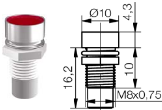
Innenreflektor mit Blendenplatte Inside Reflector With Cover Typ / type
