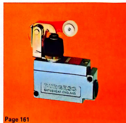
Type 9 roller-lever actuator
