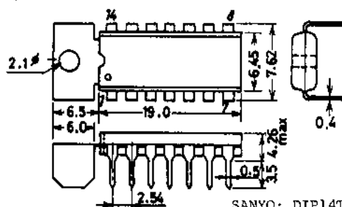
外形図 3005A-D14TIC (unit: mm)
