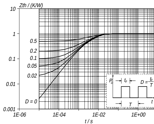
Fig.16. Transient thermal impedance. Z_{th\ j-mb} = f(t) ; parameter D = t_p/T
