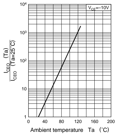
I_{CEO} - T_a
