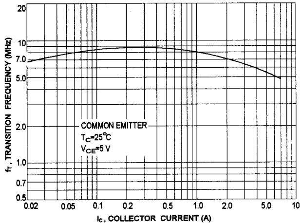
f_T - I_c
